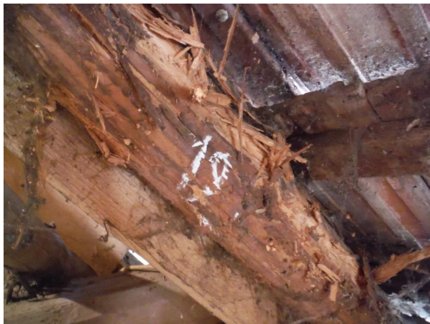
14. felvétel: Délnyugati tetősík – 19. szarufa
