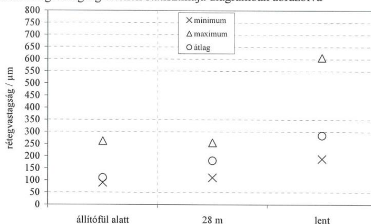
1. ábra A mért rétegvastagság értékek statisztikája diagramban ábrázolva
